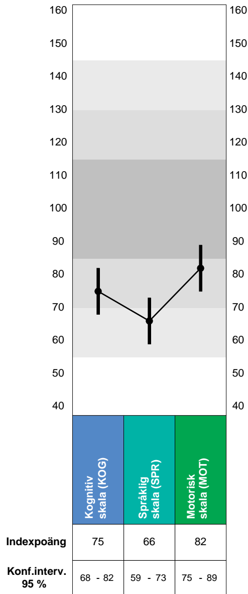
Profil över indexpoäng
