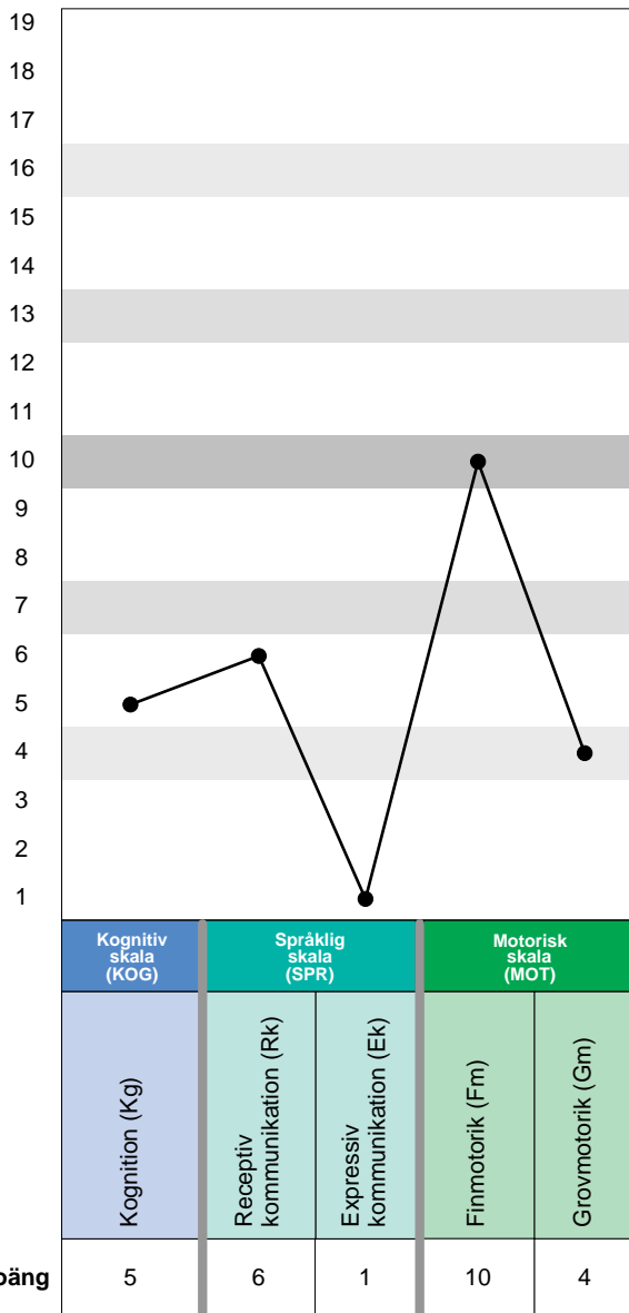
Profil över skalpoäng
